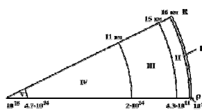
Рис. 1. Сечение нейтронной звезды массой 1.5M_{\odot} и радиусом R = 16 км. Указана плотность \rho в г/см 3 в различных частях звезды.
